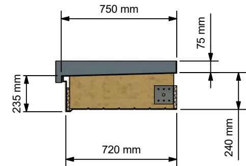
A-A ( 1 : 25 )
