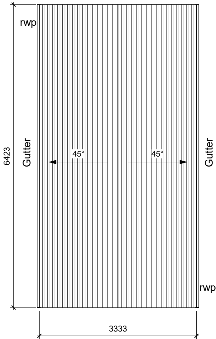
Roof Plan 1 : 50
