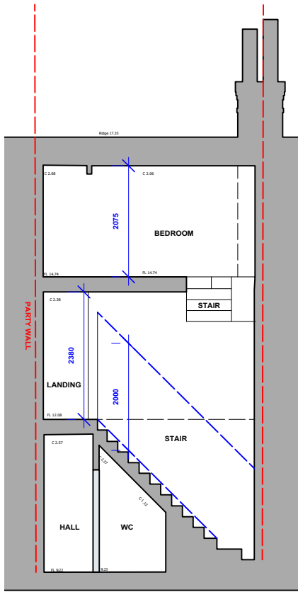
1 Section A-A
