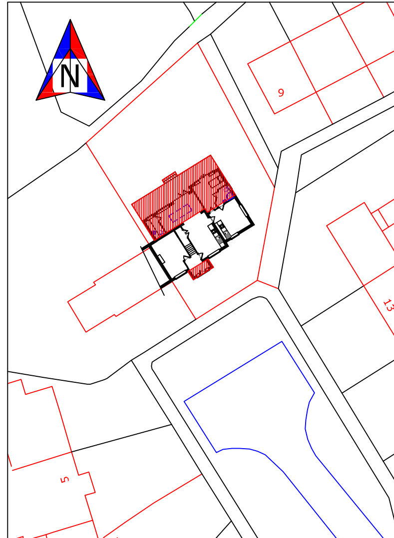
SITE PLAN 1:500
