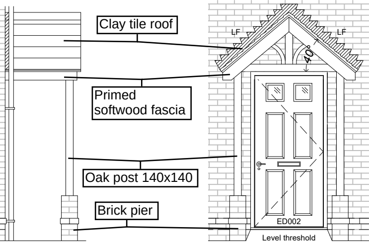
HT 2 Woodland Edge
