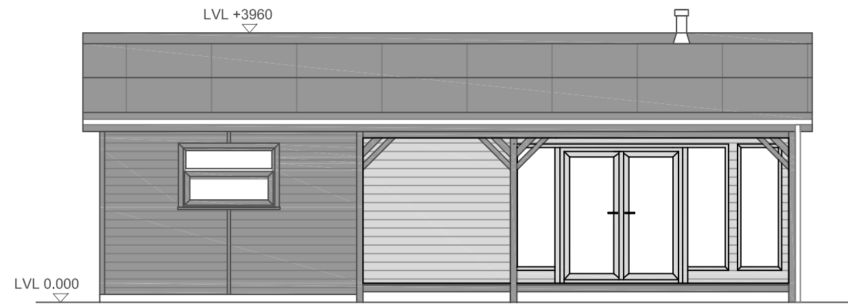
Front Elevation 1:75 A3
