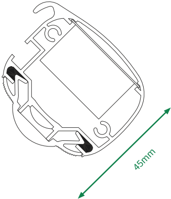
Trough Light Bracket Detail Ecolux Mini
