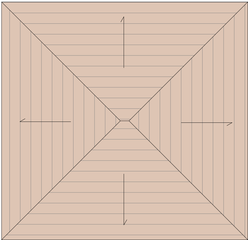
6 Roof Plan - 1 : 50
