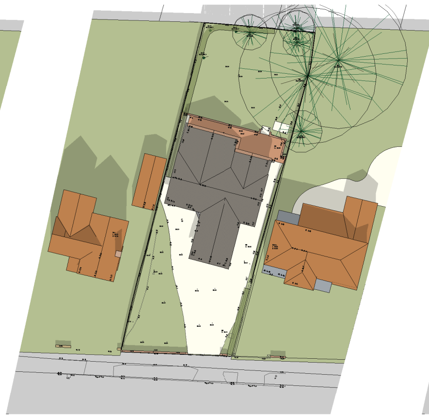
2 Existing - Autumnal Equinox 1200 1 : 500
