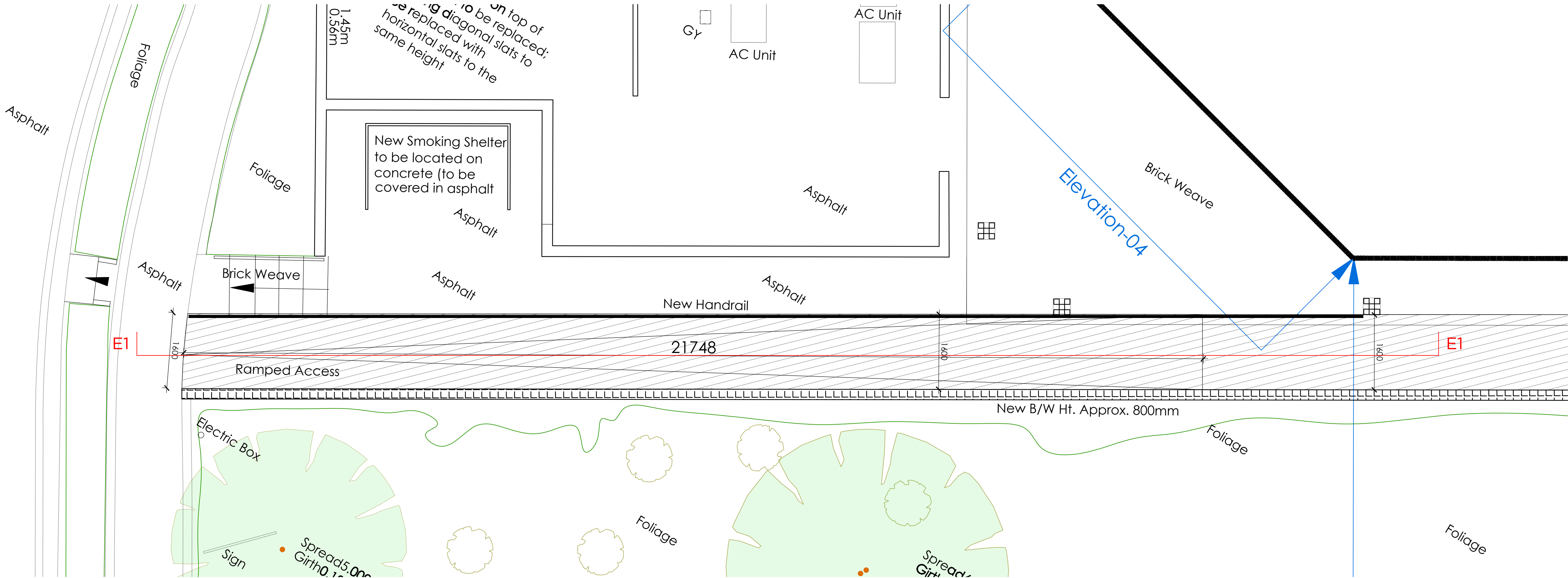
1:100 PLAN
