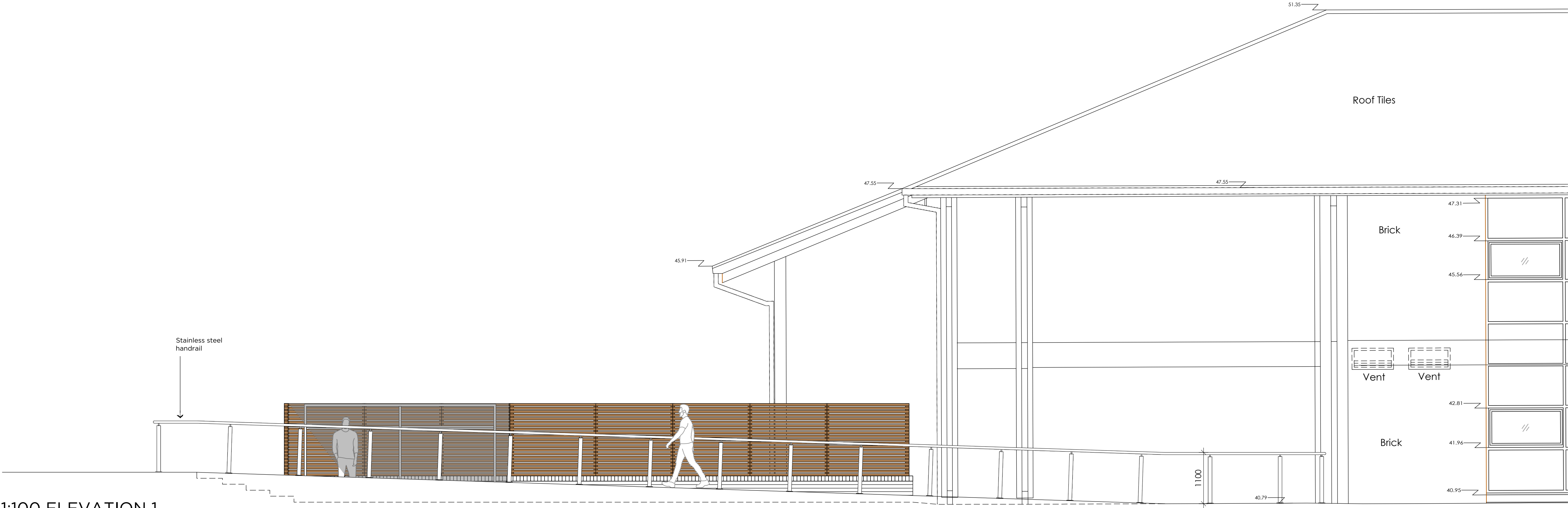
1:100 ELEVATION 1
