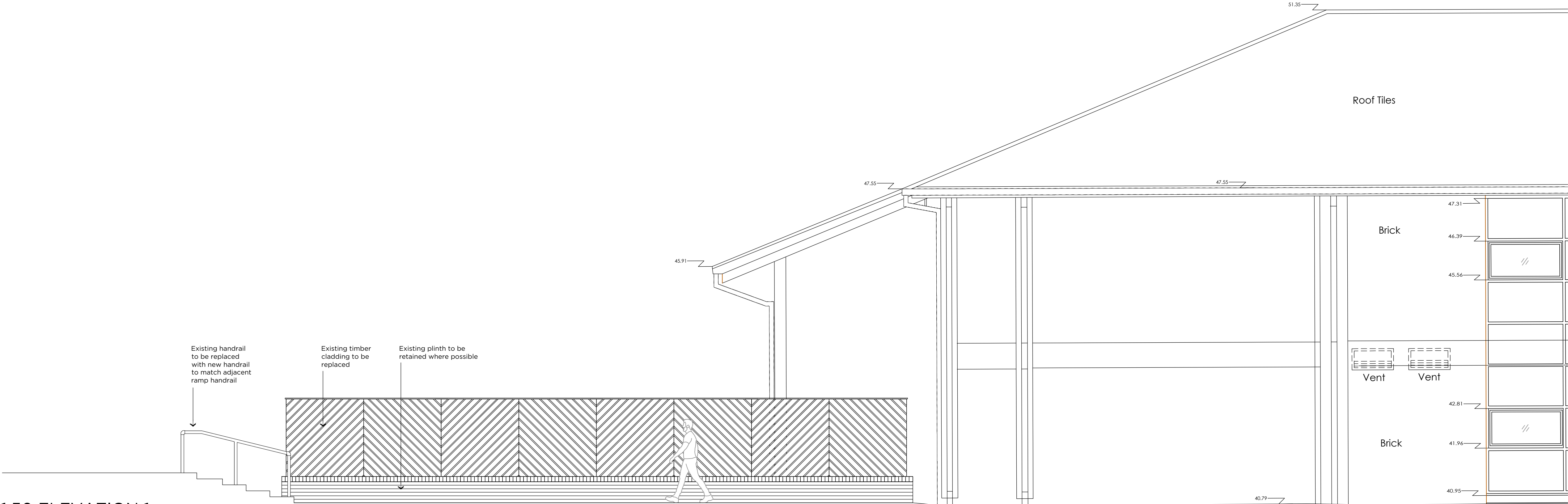
1:50 ELEVATION 1
