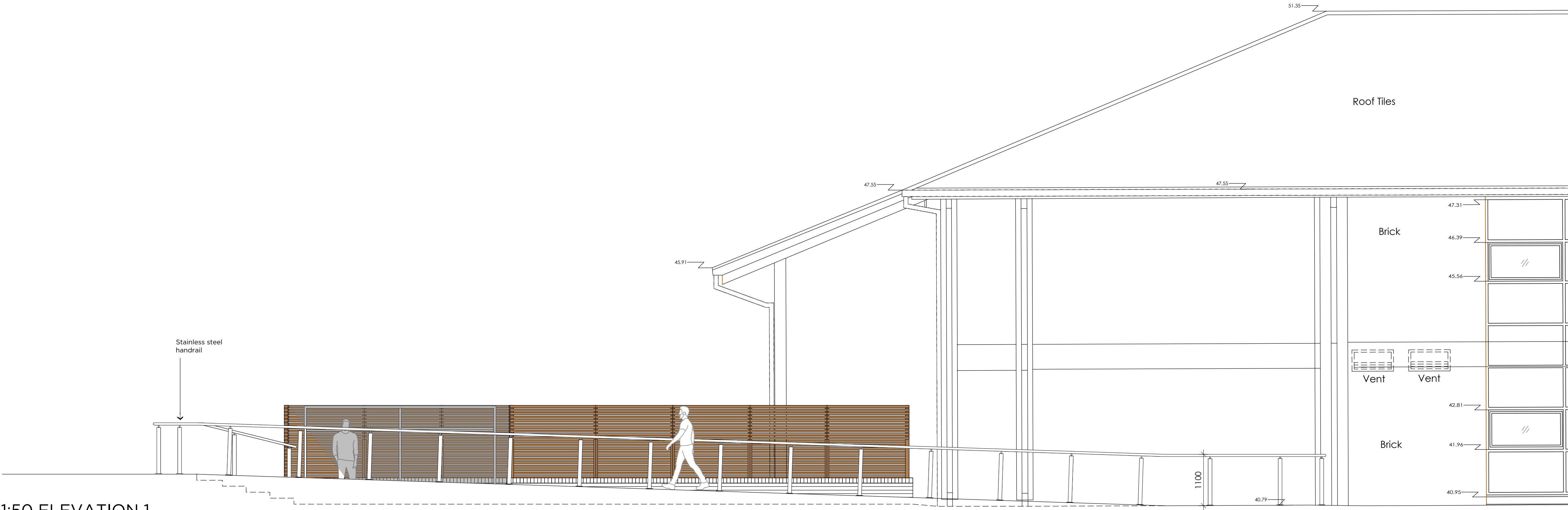
1:50 ELEVATION 1
