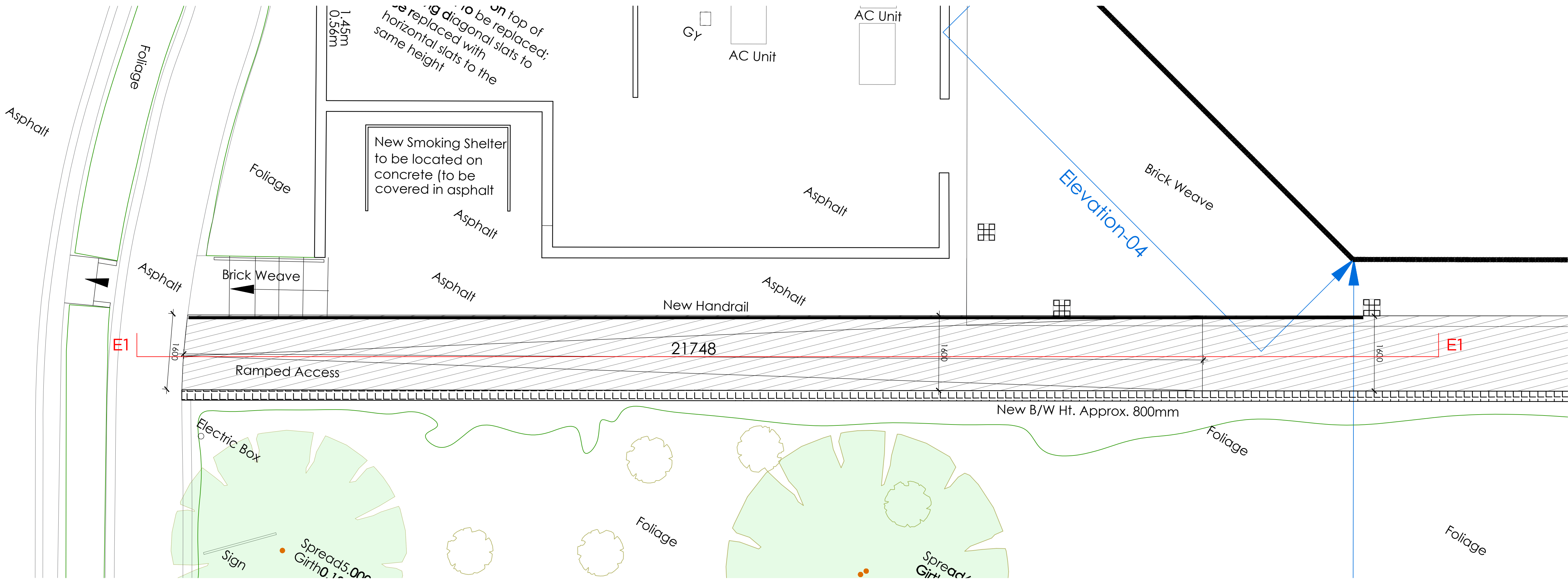
1:50 PLAN
