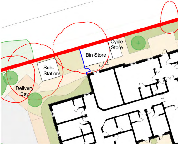
Site Plan 1 : 500
