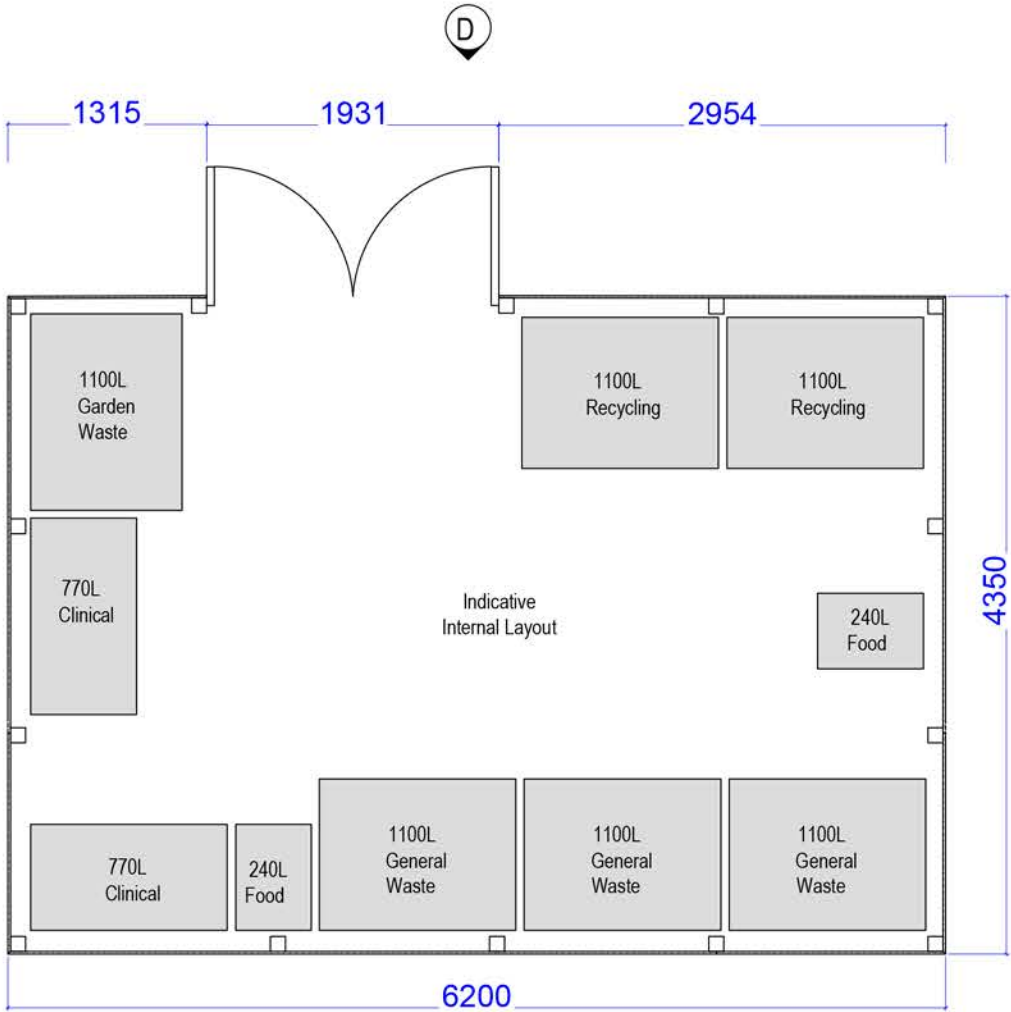
Plan 1 : 50
