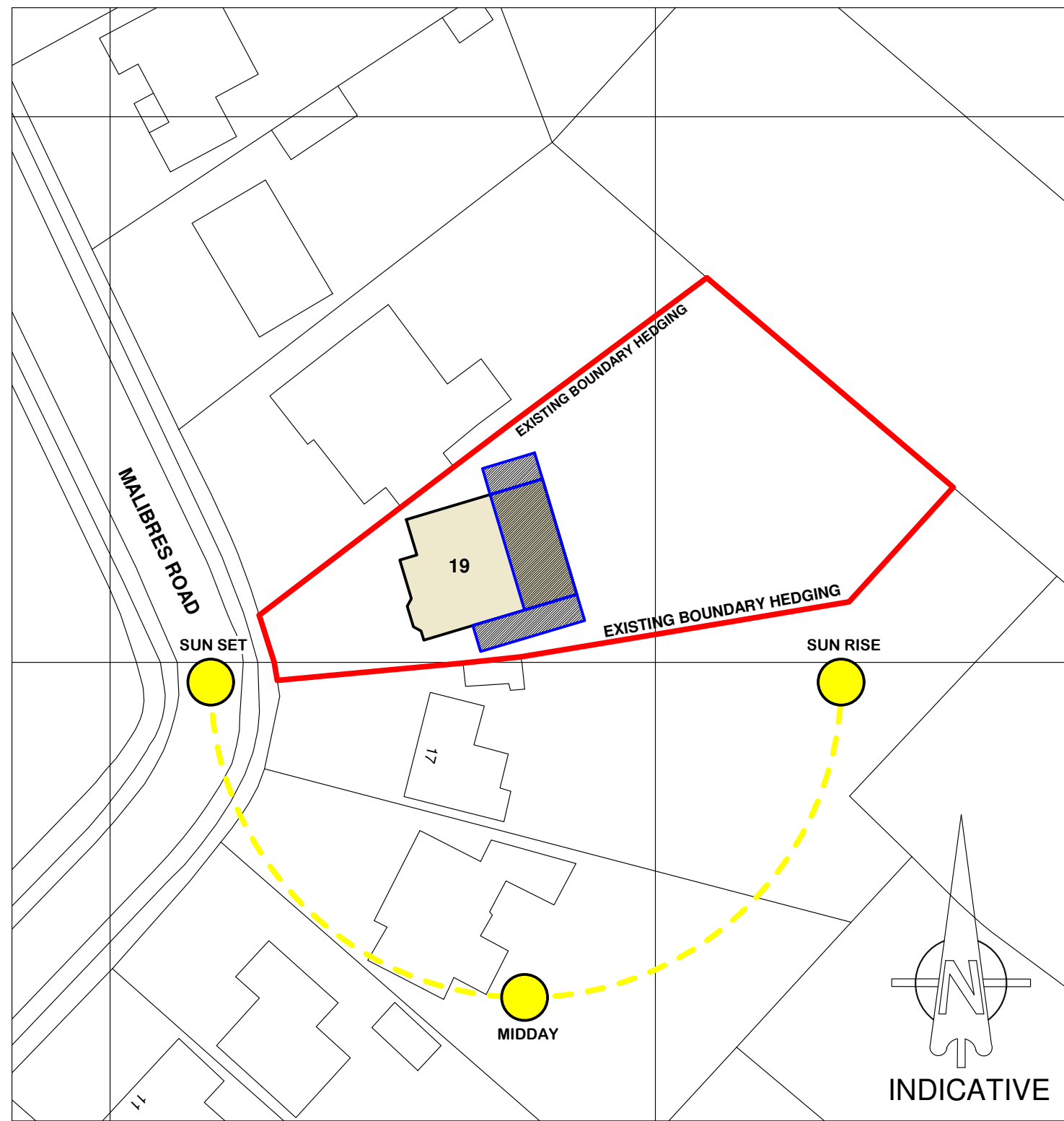
Site Plan 1:500
