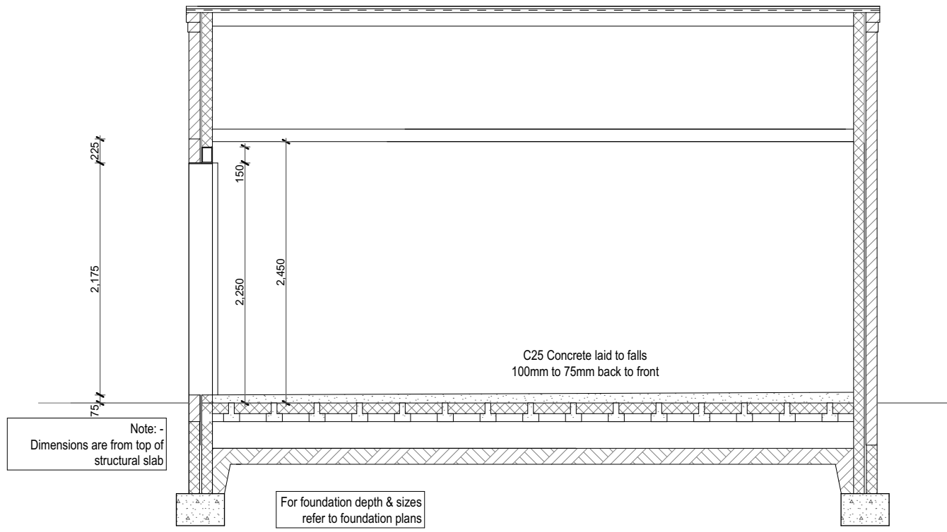
Section A-A | 1:50
