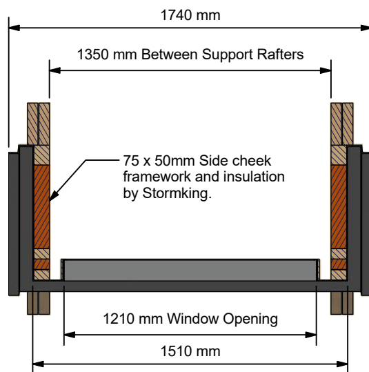
B-B ( 1:25 )
