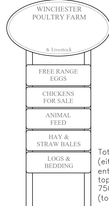
SIGNAGE 1:25
