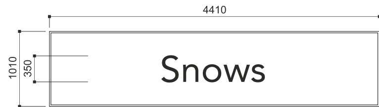
A 2No. 4410x1010 Dealername Fascias - MEDIUM
