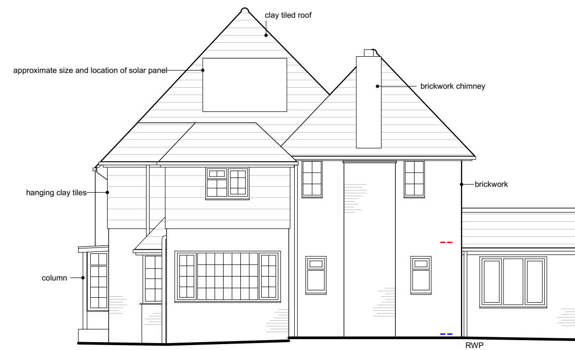
FLANK 2 ELEVATION
