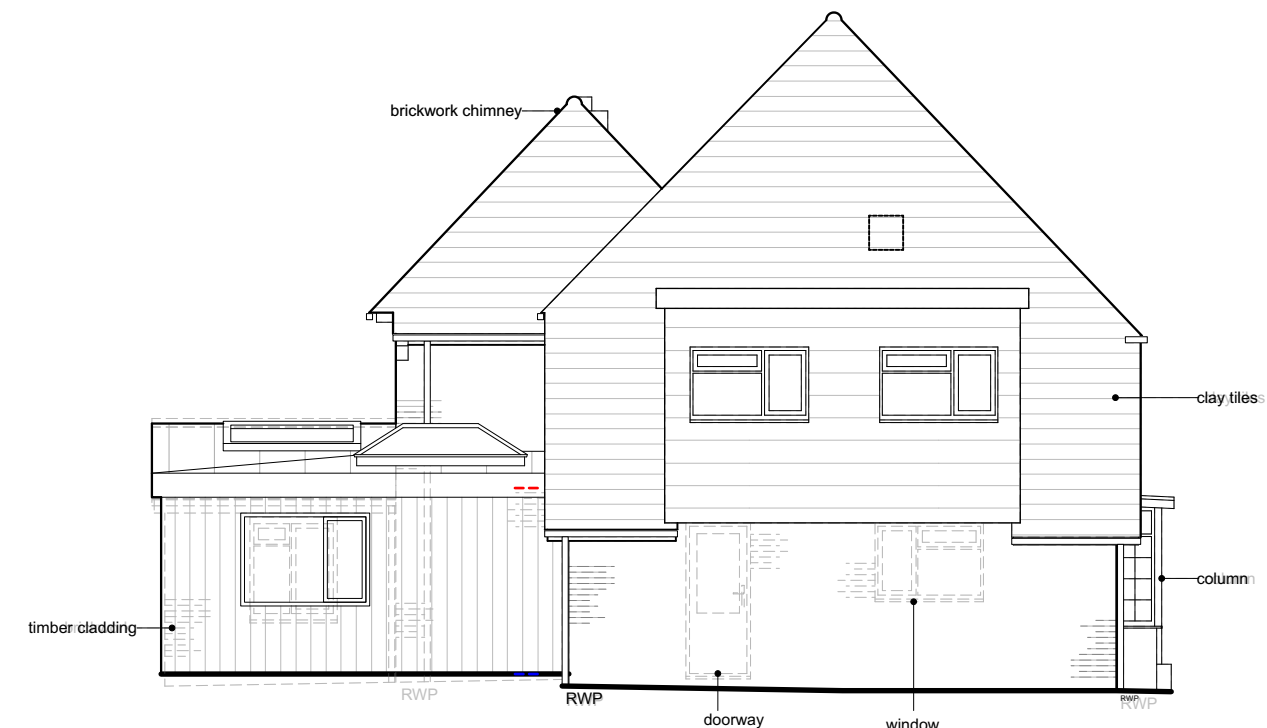
FLANK ELEVATION
