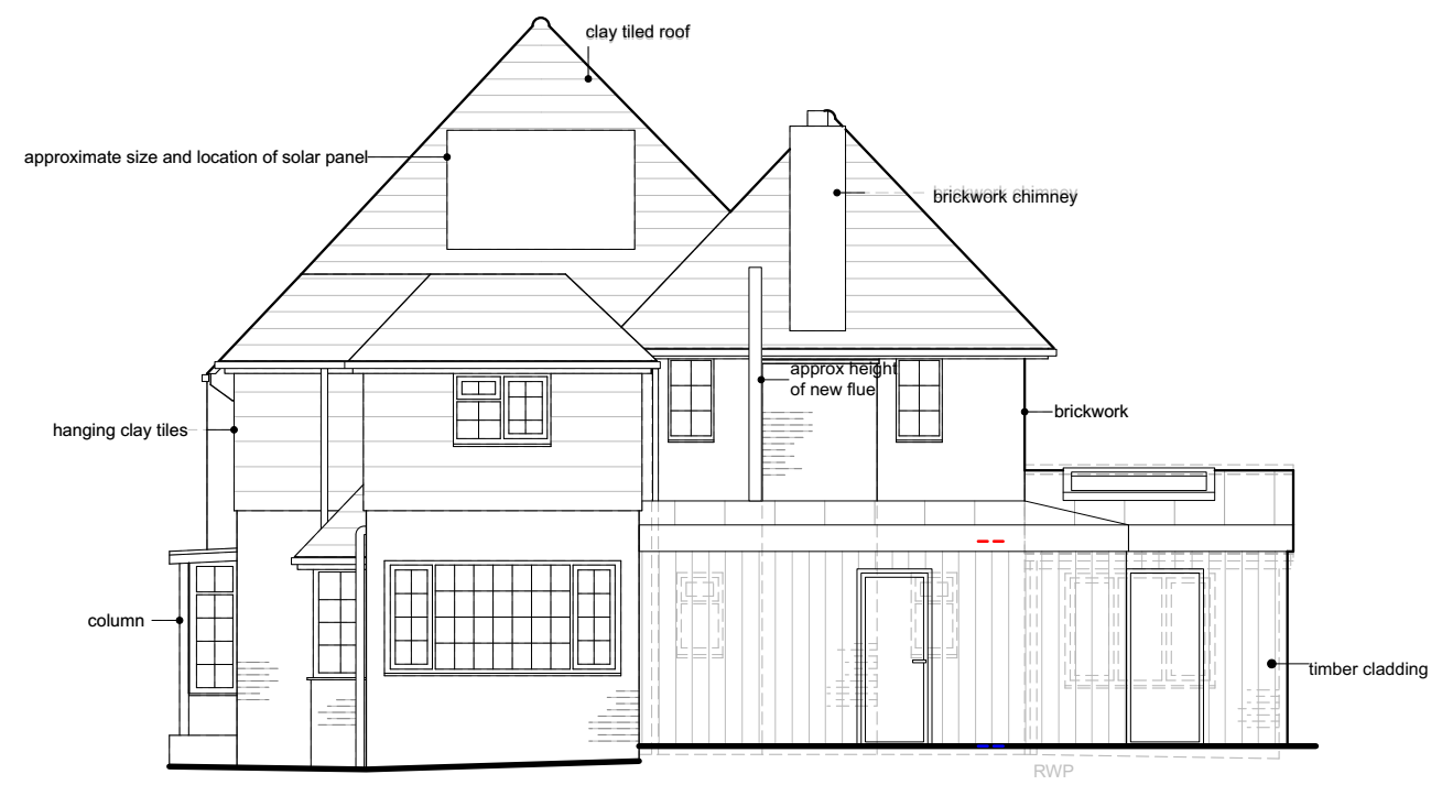
FLANK 2 ELEVATION
