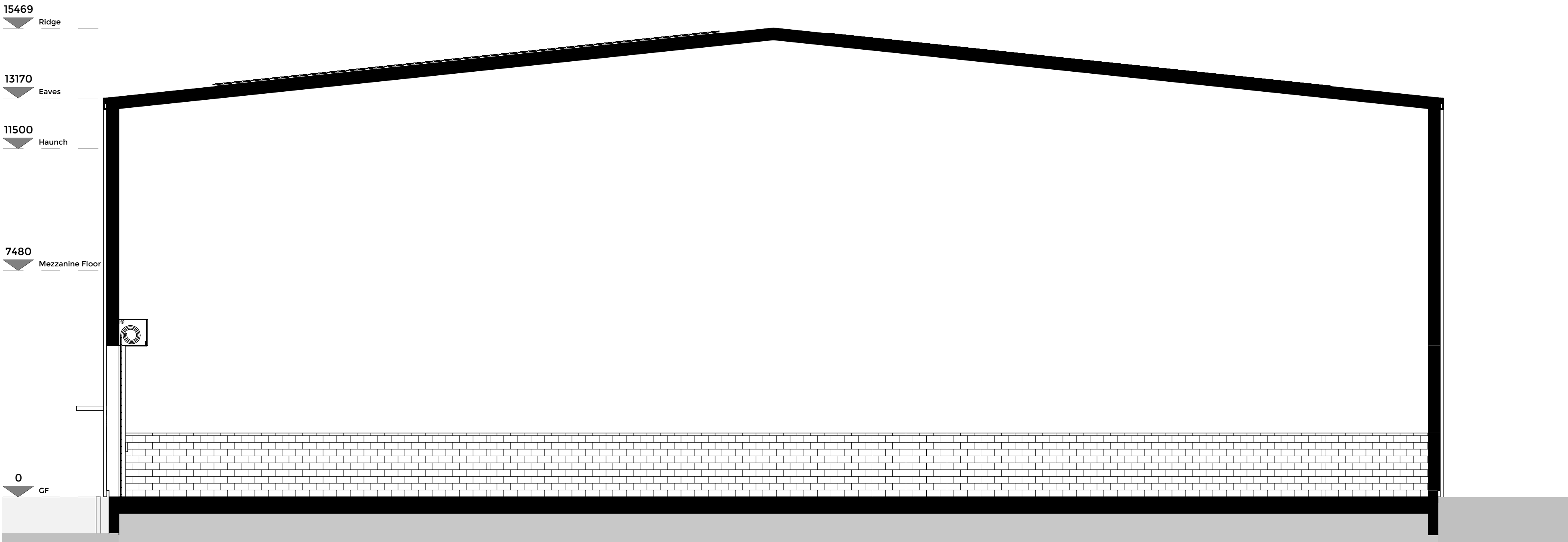
Section 2 B11 1 : 100
