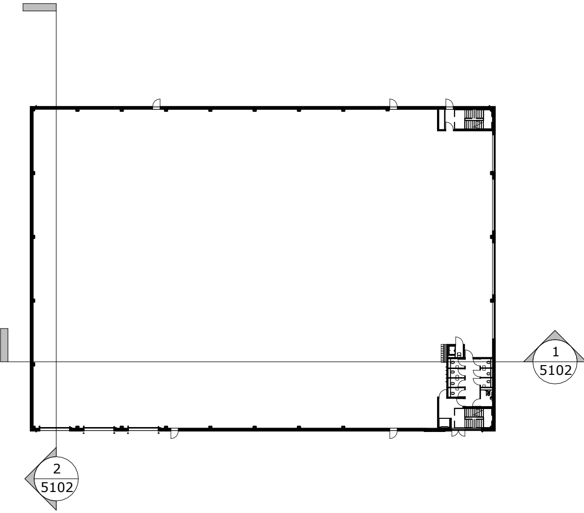
Section Key Plan 1 : 500
