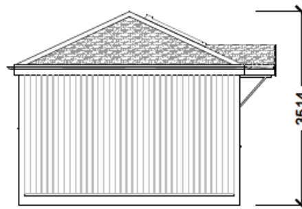
ELEVATION B
