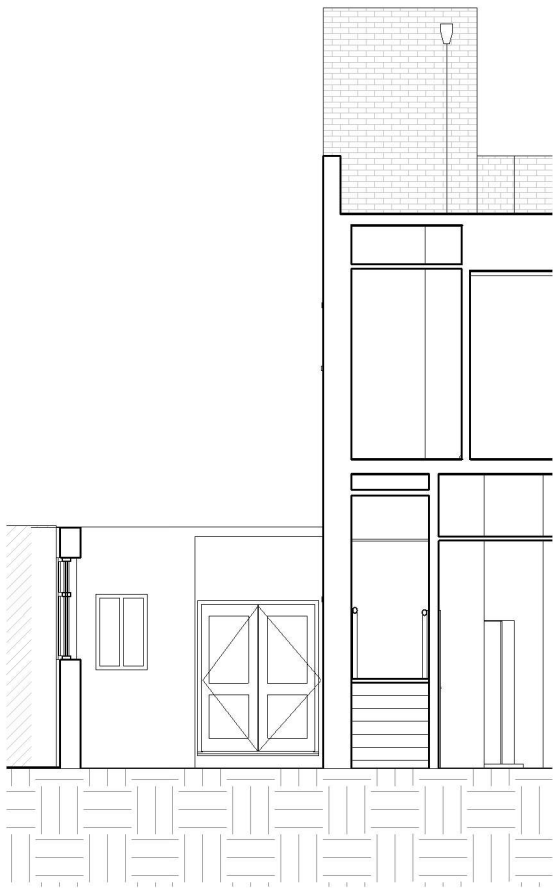
D-D 1 : 100
