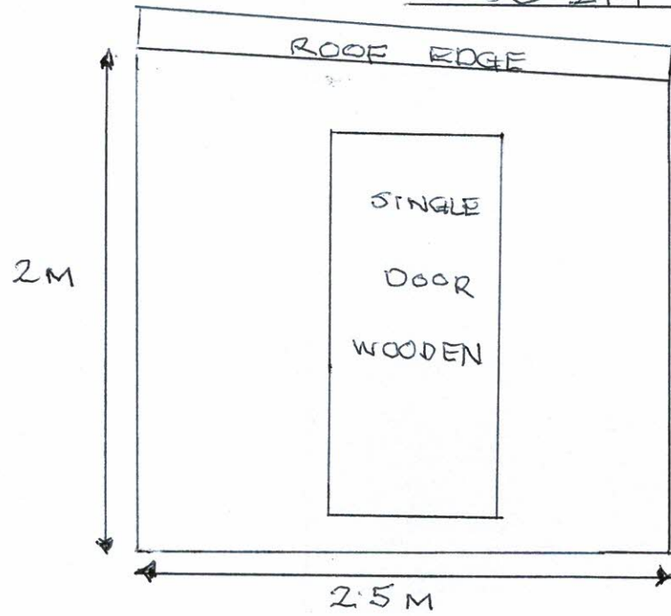
RIGHT ELEVATION
