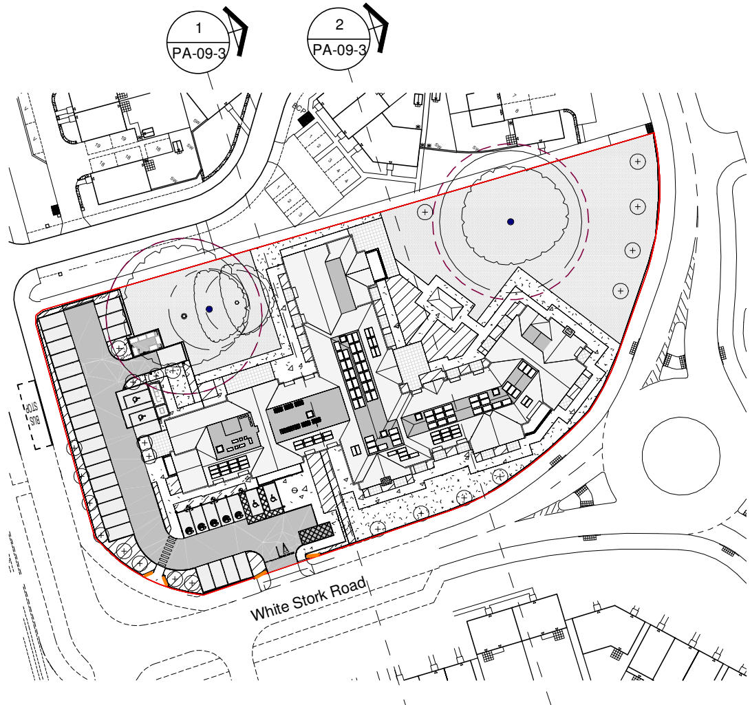
3 Site Plan 1-1000 1 : 1000
