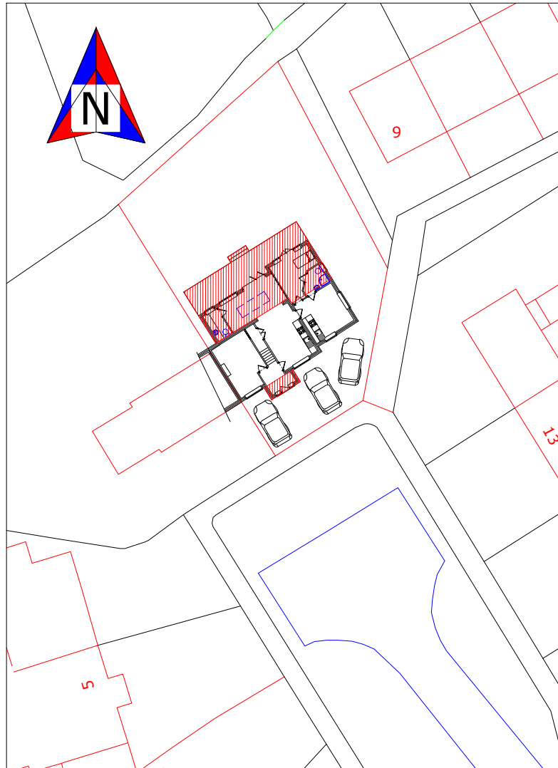
SITE PLAN 1:500
