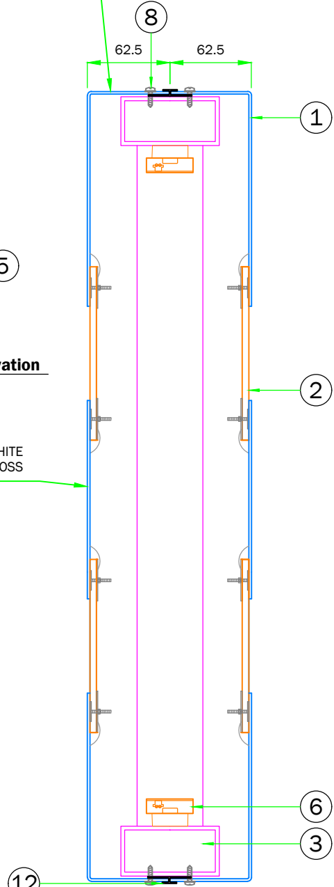
Section A-A scale 1:4
