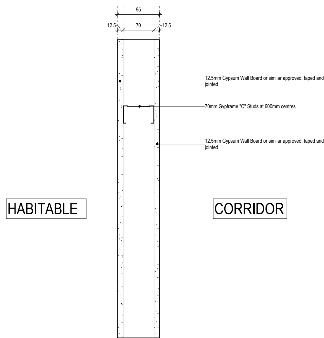
AC1_95_Stud_2x Plasterboard_30min FR
