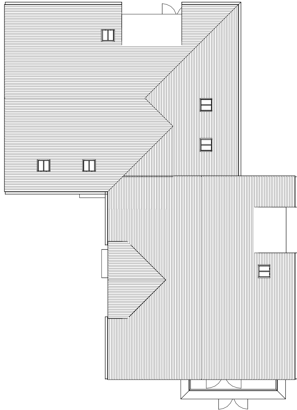
3 4 Roof Plan 1 : 100
