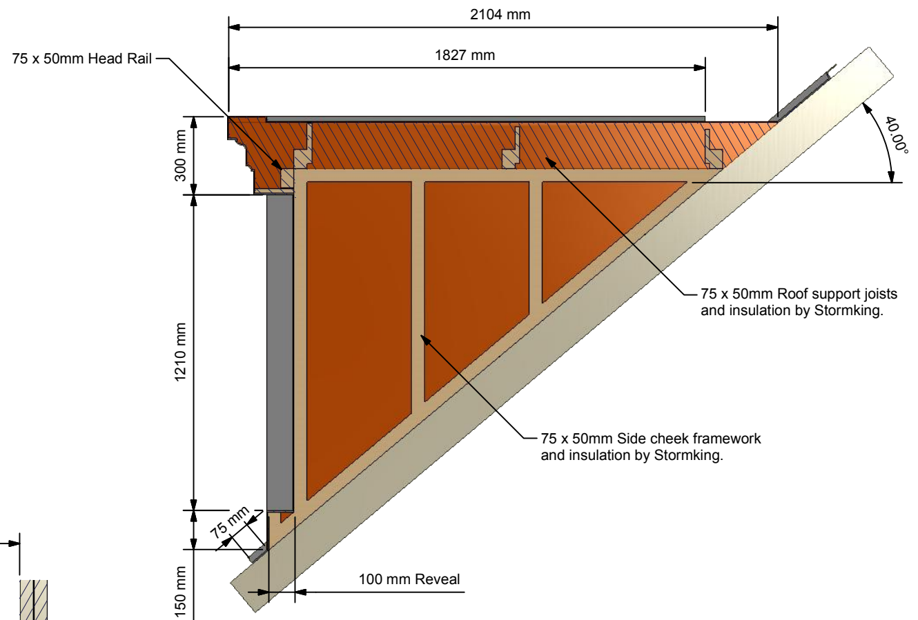
A-A ( 1:20 )
