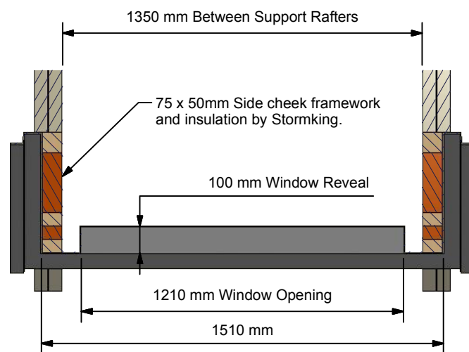
B-B ( 1:20 )
