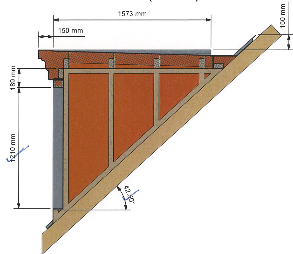
A-A ( 1 : 25 )
