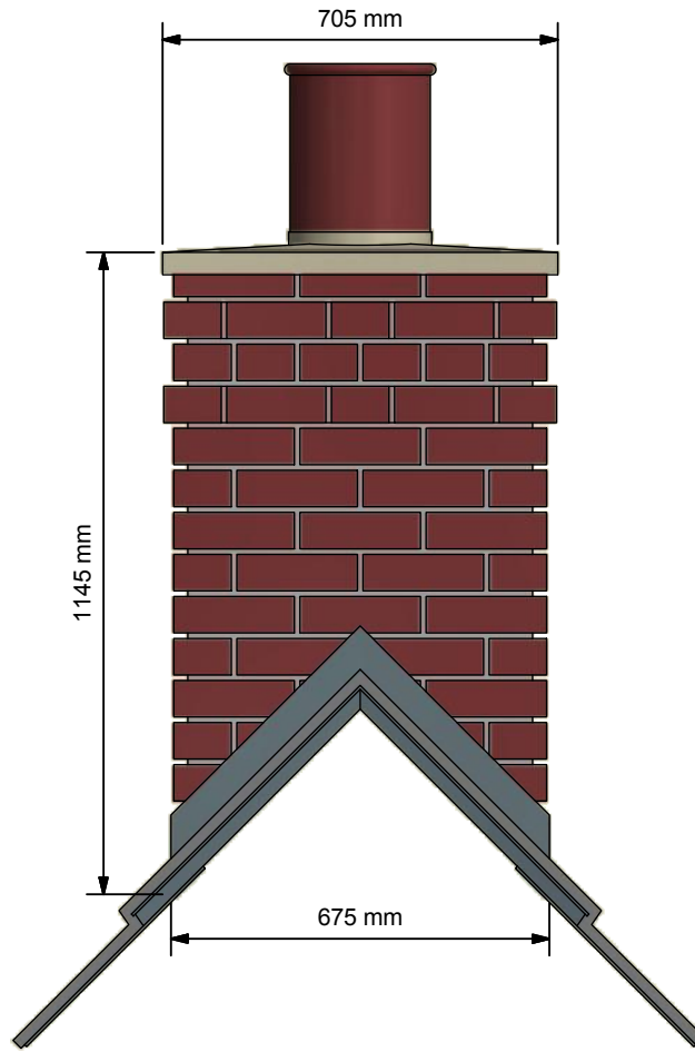
Side Elevation ( 1:15 )
