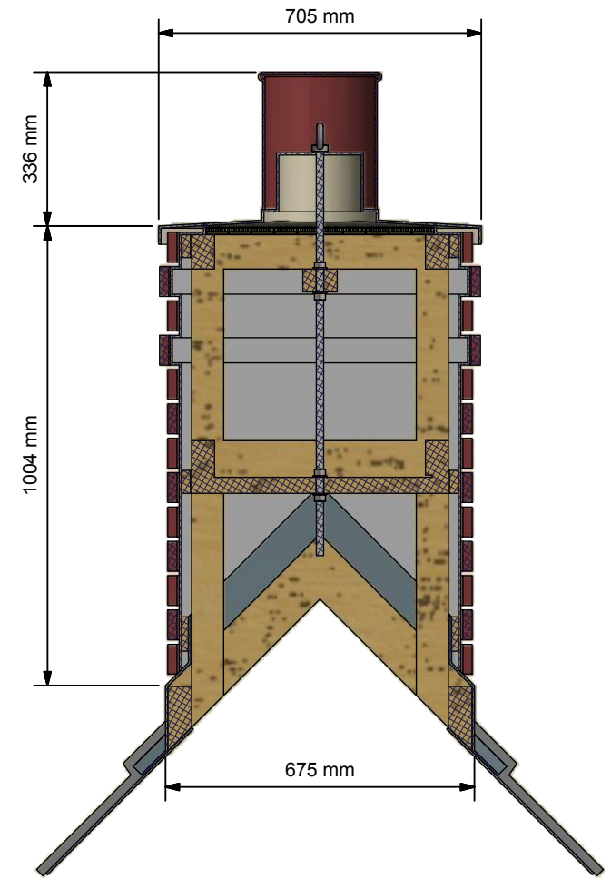
Section A-A ( 1:15 )
