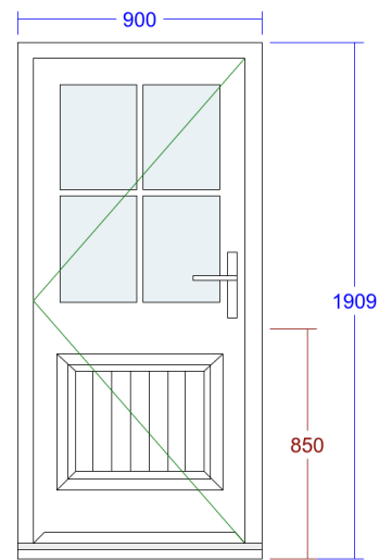
14. Entrance Door (Kitchen door )
