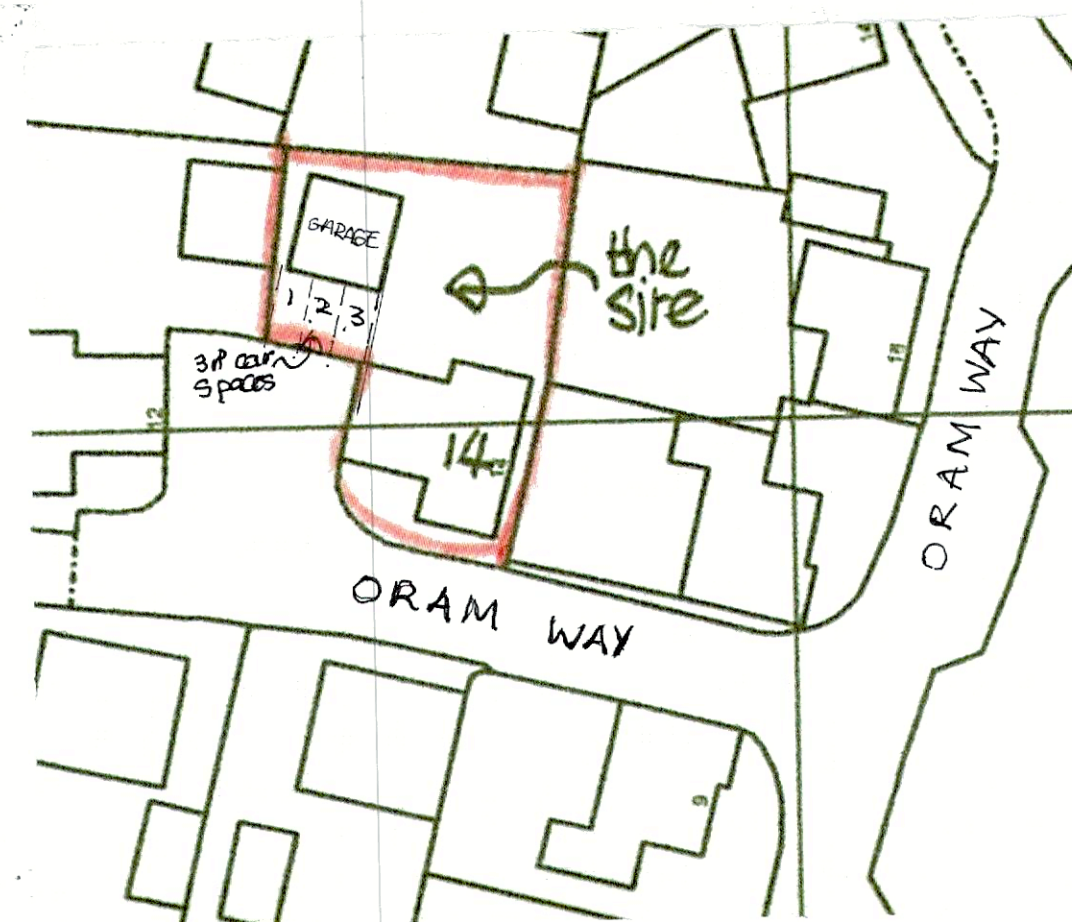
site plan 1:500
