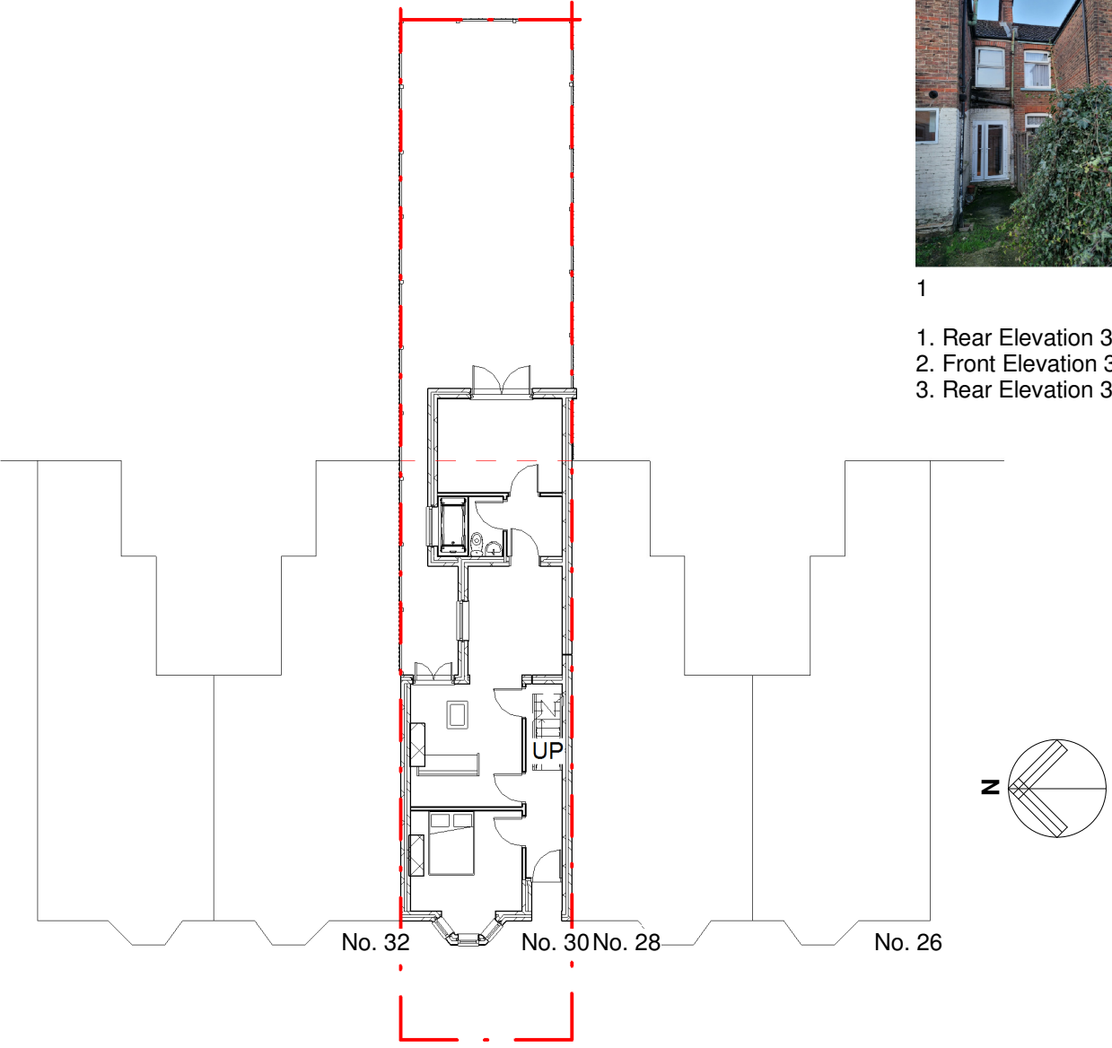
Site plan NH 1 : 200
