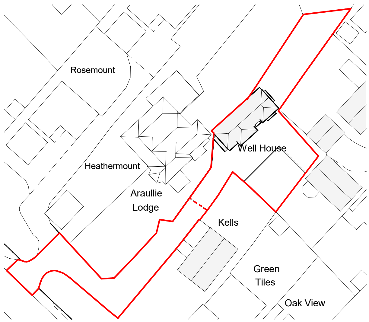
2 Site Plan 1 : 500
