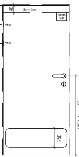
Door Elevation
