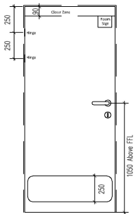
Door Elevation
