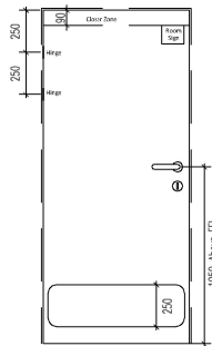
Door Elevation
