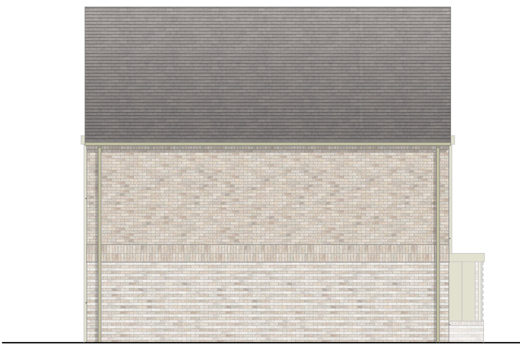
E.25-02 HGT 25 - Elevation 02 1:100
