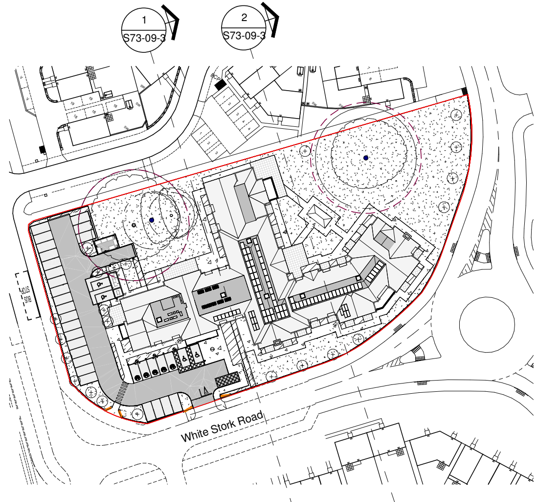
3 Site Plan 1-1000 1 : 1000
