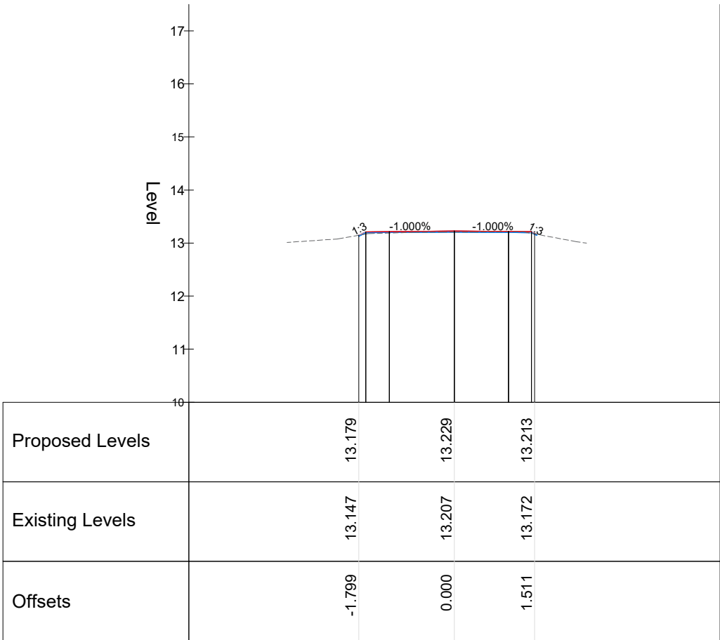
Chainage 65.000
