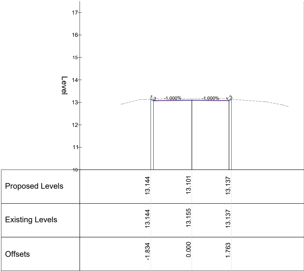
Chainage 60.000
