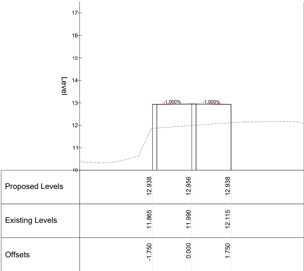
Chainage 50.000
