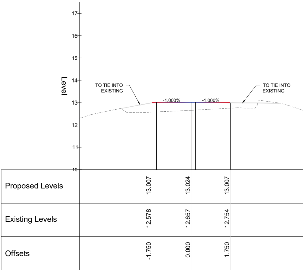
Chainage 55.000
