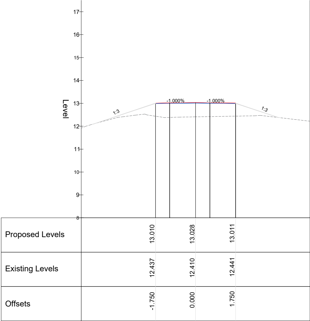
Chainage 45.000
