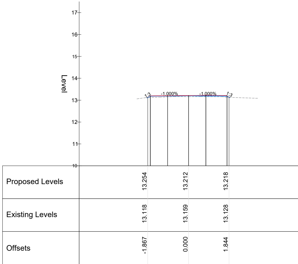
Chainage 35.000
