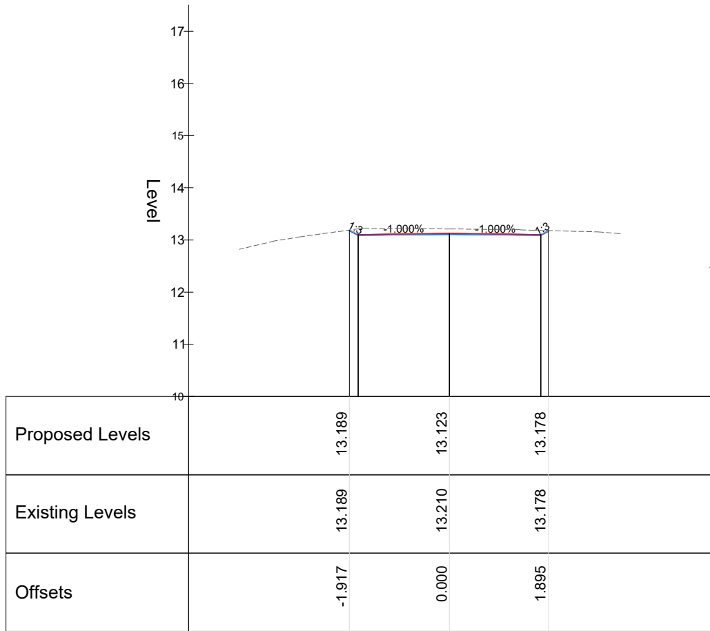
Chainage 40.000
