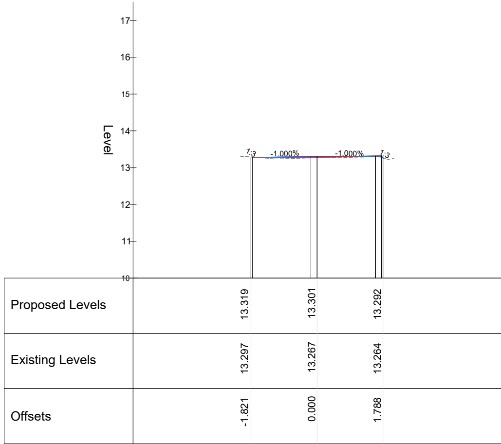
Chainage 30.000
